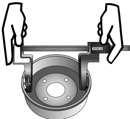
Micrómetro de Interiores indicando la lectura del diámetro del tambor.
