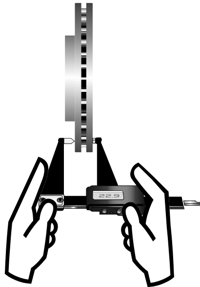
Micrómetro indicando la lectura del espesor de disco
